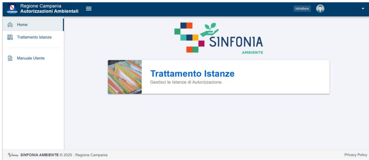
Figura 3 – Homepage piattaforma
